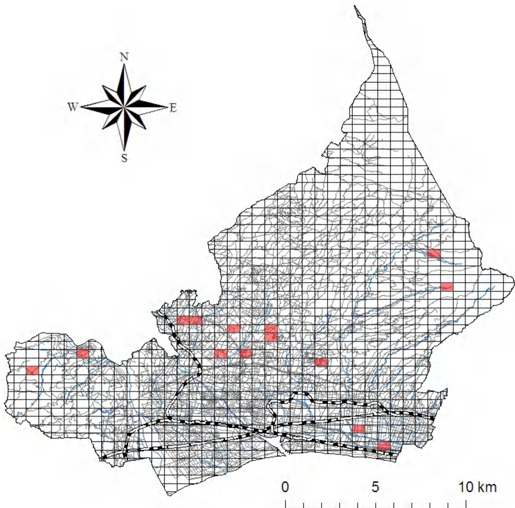
カナヘビを確認したメッシュ
